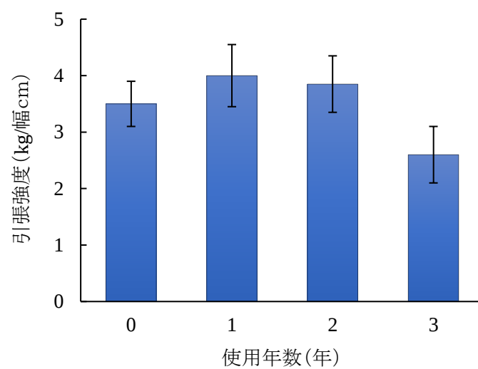
第 3-3-8 図 使用年数が新規保護材の外装の引張強度に及ぼす影響 バーは標準偏差
