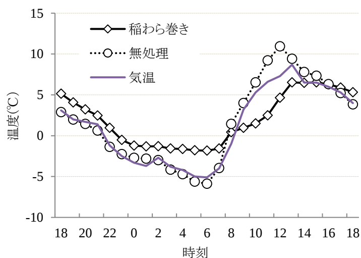
第3-3-2図 主幹部への稲わら巻きがモモ‘清水白桃’若木の主幹部温度に及ぼす影響 (主幹部南側，2012年2月27～28日)
