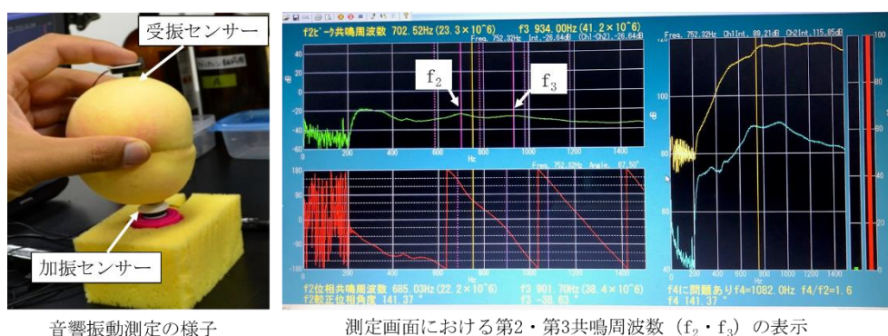
第2-7-1 図 音響振動法によるモモ果実での測定の様子（左）と測定画面における共鳴周波数の表示（右）
