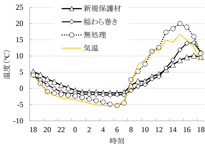
第 3-3-5 図 主幹部に巻き付けた保温資材の違いがモモ ‘清水白桃’若木の主幹部温度に及ぼす影響 (主幹部南側, 2013 年 3 月 14 日～15 日)
