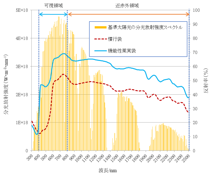
第 2-2-6 図 機能性果実袋と慣行袋の分光反射率の違い 基準太陽光の分光放射強度スペクトルは、 ISO 9845-1:1992 を参照し作成
