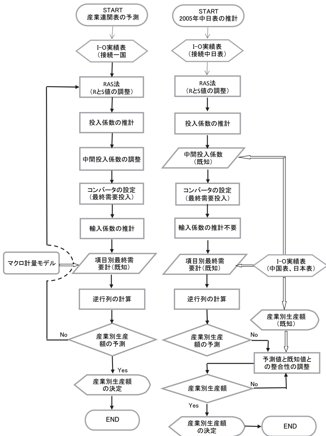
図表 1 作業のフローチャート：Econamate I-O による産業連関表の予測 VS 2005 年中日表の推計
